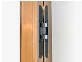
618 Maalattu oksaton tiivistetty puukarmi piilosaranoilla karmisyvyys 92 mm. Myydään vain settinä tiettyjen ovimallien kanssa. Ovi suorareunainen. Koot 7-10 x 21M ja pariövet 13, 15 x 21M
